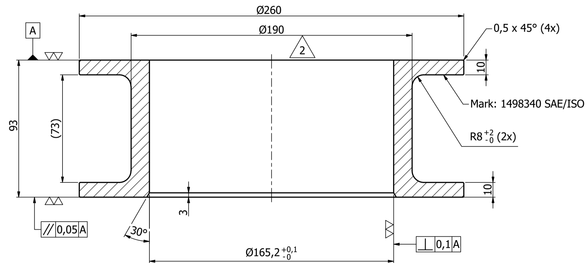
A-A ( 1 : 1,5 )
