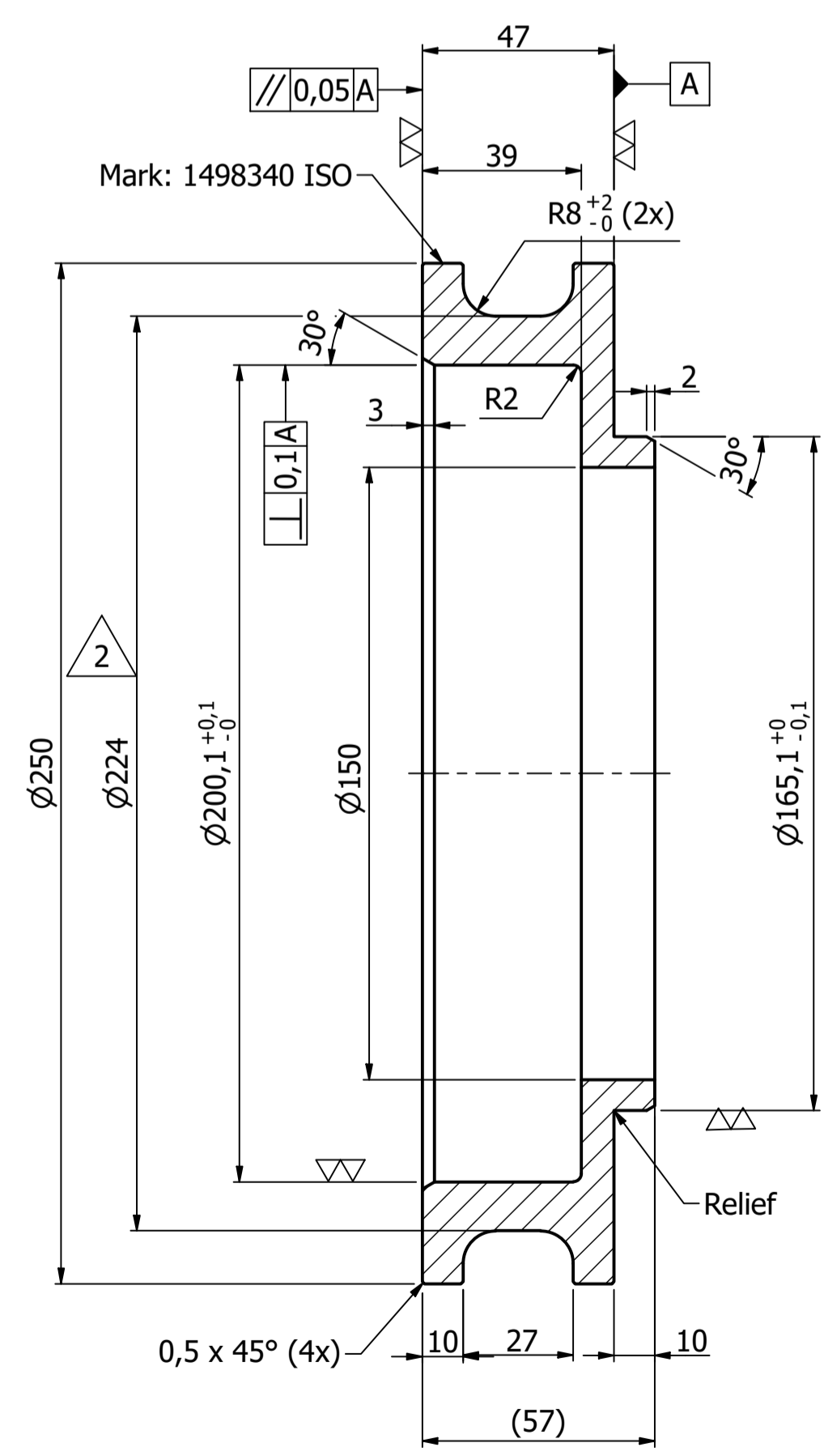
B-B ( 1 : 1,5 )
